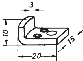
Cu-versilbert Bestell-Nr. A1340 m. Ag-Aufl. u. vers. Bestell-Nr. A1340 Ag
