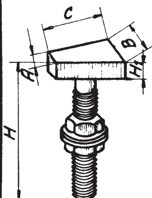
Messingkopf mit Messingscheiben und Messingmuttern
