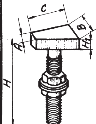
Messingkopf mit Messingscheiben und Messingmuttern
