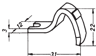
Cu-versilbert Bestell-Nr. A1340 m. Ag-Aufl. u. vers. Bestell-Nr. A1340 Ag
