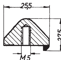
Bestell-Nr. A78 ....mm breit
