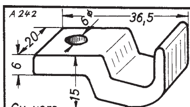
A 242 Cu vers. Bestell-Nr. A 242 m. Silberaufl. u. versilbert Bestell-Nr. A 242 Ag
