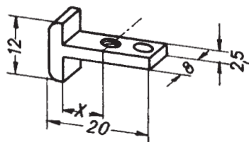
X = 5 Bestell-Nr. A 555 X = 7,5 Bestell-Nr. A 555 a
