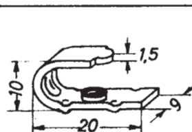
Bestell-Nr. A540 L
