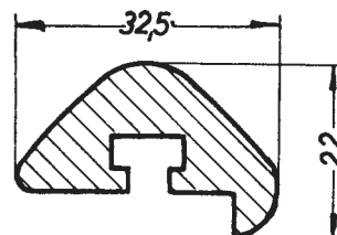
Bestell-Nr. A80 ....mm breit
