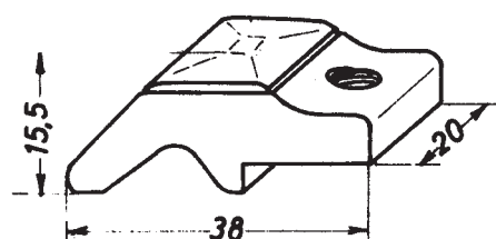
Bestell-Nr. A 77/20 Ag
