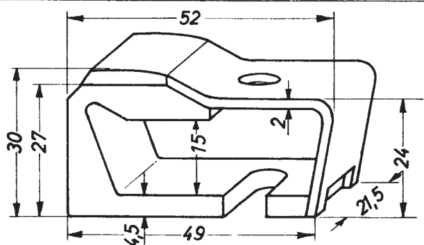
Bestell-Nr. A 337 N
