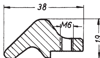
Bestell-Nr. A77 ....mm breit
