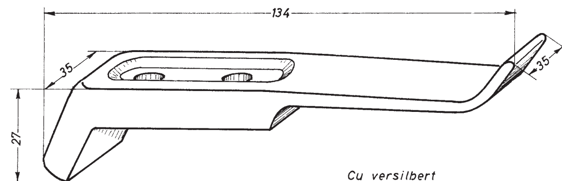
A 867 Cu versilbert Bestell-Nr. A 867 m. Silberaufl. u. versilbert Bestell-Nr. A 867 Ag H = 28 Cu versilbert Bestell-Nr. A 867 a m. Silberaufl. u. versilbert Bestell-Nr. A 867 a Ag H = 38
