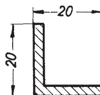
Bestell-Nr. A68 ....mm breit
