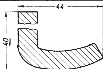
Bestell-Nr. A62 ....mm breit
